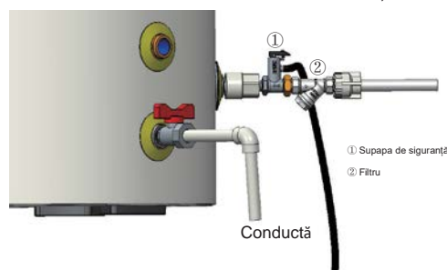
Modul 1 de instalare a supapei de siguranță pentru conducta de apă de la robinet (presiunea apei la intrare = 0,1 ~ 0,5MPa)
