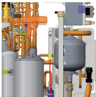
Supapa de încărcare 1
