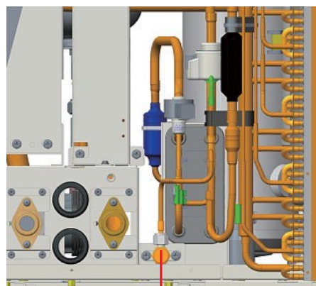
Supapa de încărcare 2
