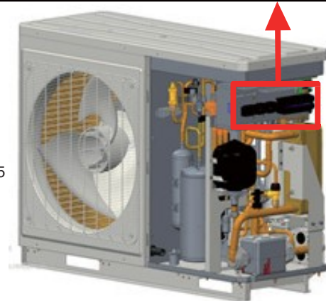
Regletă de borne XT5
