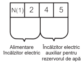
Placa cu borne XT4
